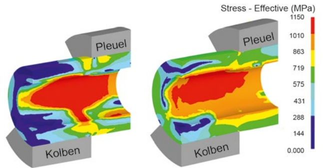
Ergebnisse der Biegebelastungssimulation eines Kolbenbolzens, links: isotropes Materialmodell; rechts: isotrop-kinematisches Materialmodell
