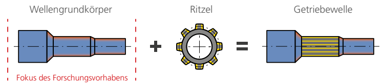
Schematische Darstellung der Herstellung einer gebauten Getriebewelle durch Fügen eines Wellengrundkörpers und eines Ritzels
