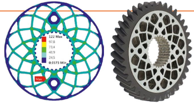
Links: Geometrie und Simulation (Ergebnisse in MPa) einer einzelnen Blechlage des blechpaketierten Radkörpers
